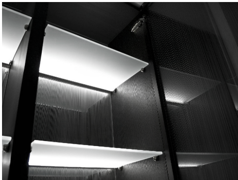
Кліпса чорна світлодіодна алюмінієва для підсвітки скляних полиць, чорний провід
